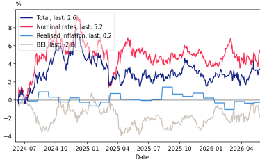
DGBi'34: Return Last 2Y, Inflation rel. to Initial BEI
